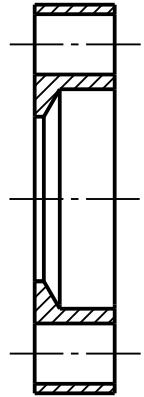
Schnitt B-B
